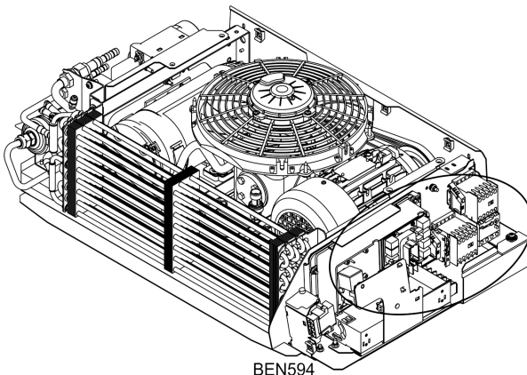
Figura 11. Posizione fusibili (coperchio del condensatore rimosso)
