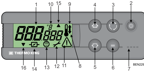
Figura 9. Display, tasti e simboli del quadro comandi in cabina (HMI)
