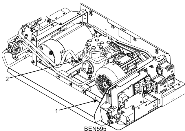
Figura 12. Posizione del numero di serie del compressore di riserva e del condensatore
