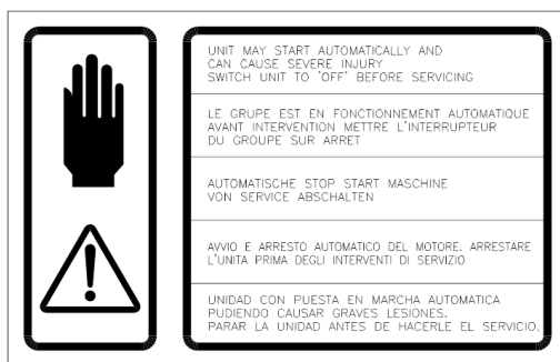
Figura 5. Avvertenza avvio automatico dell'unità
